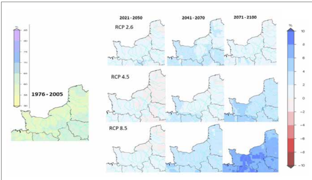
FIGURE 12 : Pourcentage des précipitations extrêmes au-dessus du 90e centile annuel selon les différents scénarios d'émissions de CO2 du GIEC et selon différents horizons (expérience Météo France CNRM 2014 : Modèle Aladin, Période de référence : 1976-2005)
