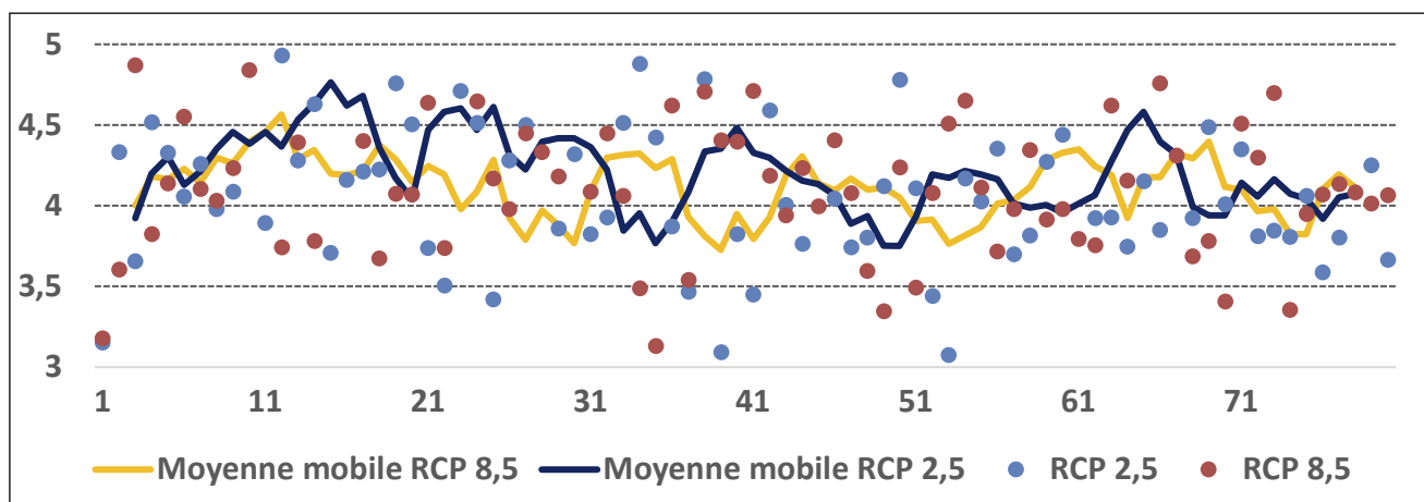
FIGURE 14 : Évolution de la vitesse moyenne du vent durant les mois d'hiver selon les scénarios extrêmes d'émission en CO 2 du GIEC (RCP 2,5 et 8,5) (expérience Météo France CNRM 2014 : Modèle Aladin, Période de référence : 1976-2005 / données issues du site DRIAS : http://www.drias-climat.fr/ )
