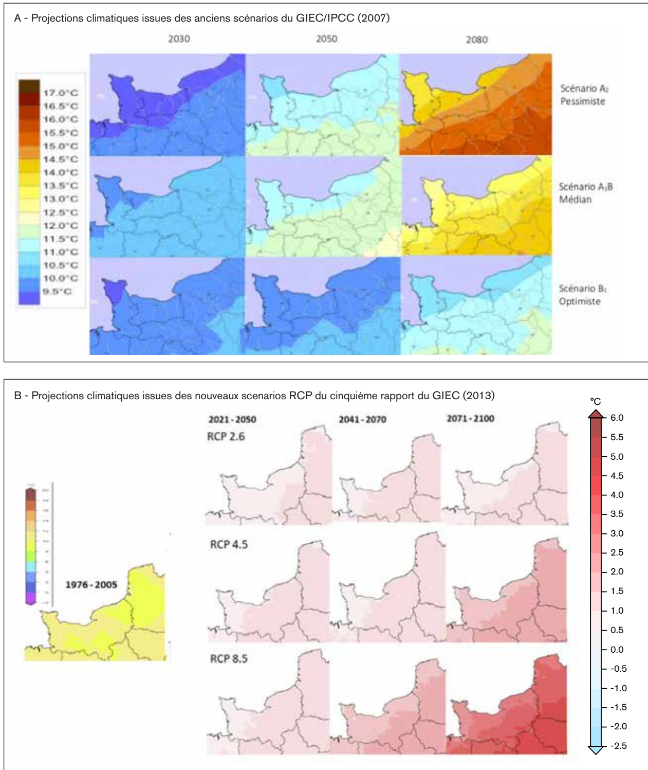
FIGURE 4 : Évolution attendue des températures moyennes annuelles en Normandie à l'horizon 2100 (sources des données : modélisation A, DREAL BN, 2010 et DREAL HN, 2011 / modélisation B : données DRIAS, 2018)
