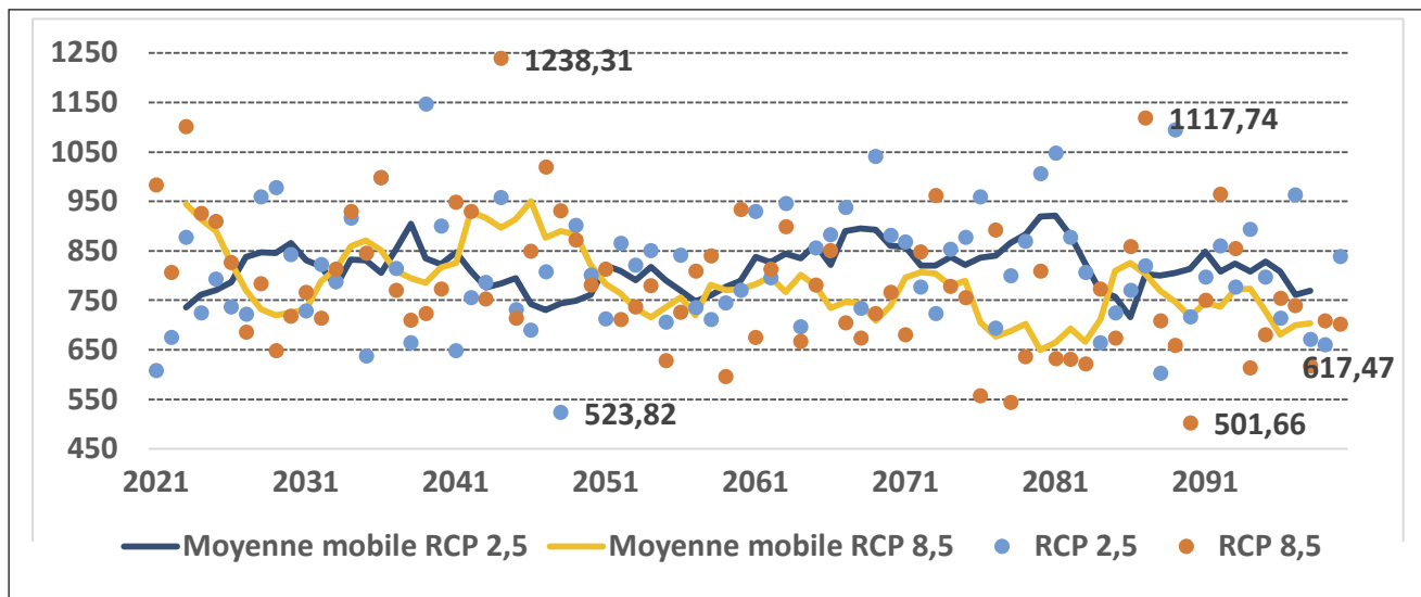
FIGURE 9 : Évolution des cumuls de pluies à Rouen selon les scénarios extrêmes d'émission en CO 2 du GIEC (RCP 2,5 et 8,5) (expérience Météo France CNRM 2014 : Modèle Aladin, Période de référence : 1976-2005 / données issues du site DRIAS : http://www.drias-climat.fr/ )
