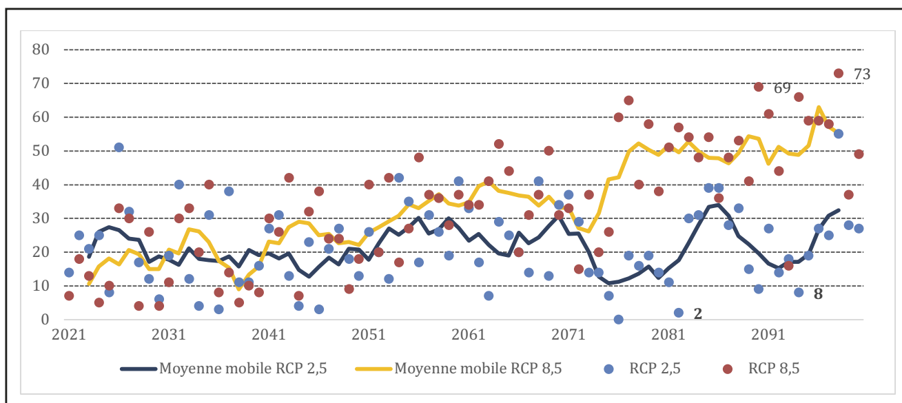
FIGURE 11 : Évolution du nombre de jours de chaleur (maximum \geq 25^{\circ}\text{C} ) à Rouen selon les scénarios extrêmes d'émission en \text{CO}_2 du GIEC (RCP 2,5 et 8,5) (expérience Météo France CNRM 2014 : Modèle Aladin, Période de référence : 1976-2005 / données issues du site DRIAS : http://www.drias-climat.fr/ )
