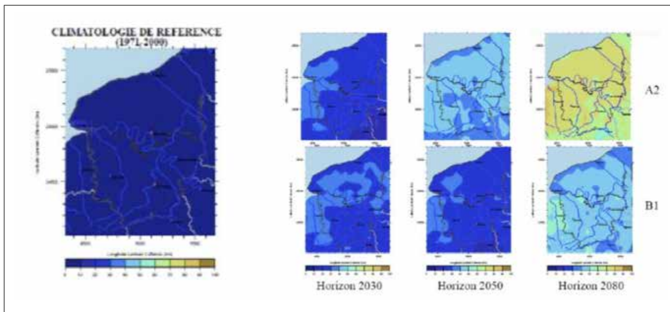
FIGURE 10 : Évolution de la sécheresse (en pourcentage) sur le territoire de l'ex Haute-Normandie aux horizons 2030, 2050 et 2080 (Source : Météo France)
