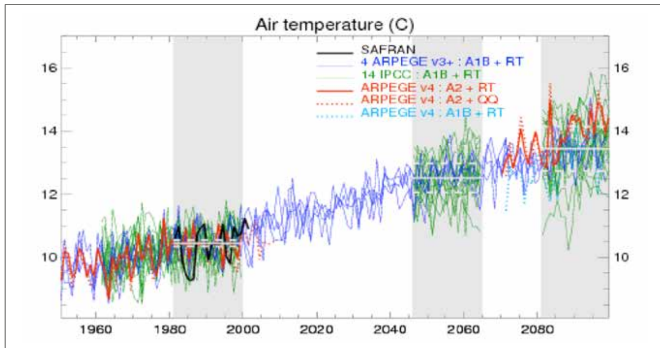
FIGURE 5 : Évolution de la température de l'air (moyennes annuelles en °C) dans le bassin de la Seine entre 1950 et 2100.
