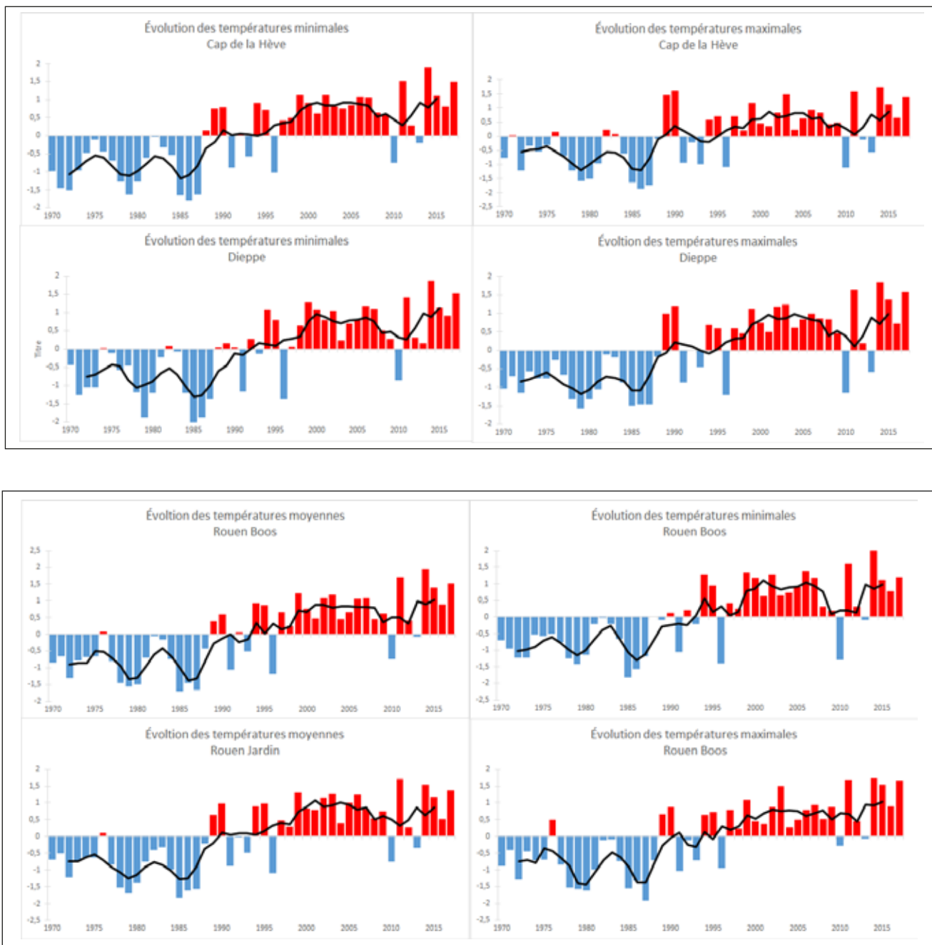
FIGURE 2 : Évolution des températures en zone urbaine (stations Rouen-Boos et Rouen-Jardin) et sur le littoral (stations de Dieppe et du Cap de la Hève), à partir du calcul d'indices centrés réduits
