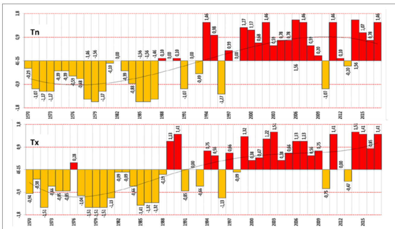
FIGURE 1 : Indice régional calculé à partir des écarts centrés réduits des températures minimales et maximales pour dix stations de l'ex région Haute-Normandie (liste des stations dans le tableau 1) – Légende : Tn : Températures minimales ; Tx : Températures maximales
