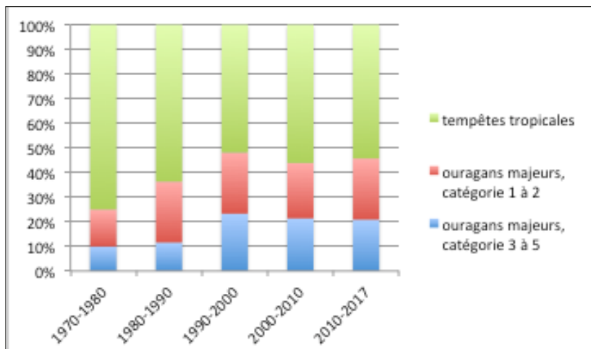
FIGURE 13 : Répartition des ouragans selon leur intensité dans le bassin nord atlantique, par décennie, en % (Source HNC-NOAA)
